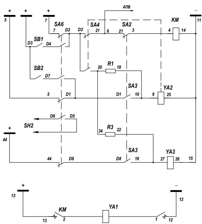
Рисунок 5. Схема электрическая соединений и принципиальная привода ПЭМ-УЭТМ®-4 УХЛ1
