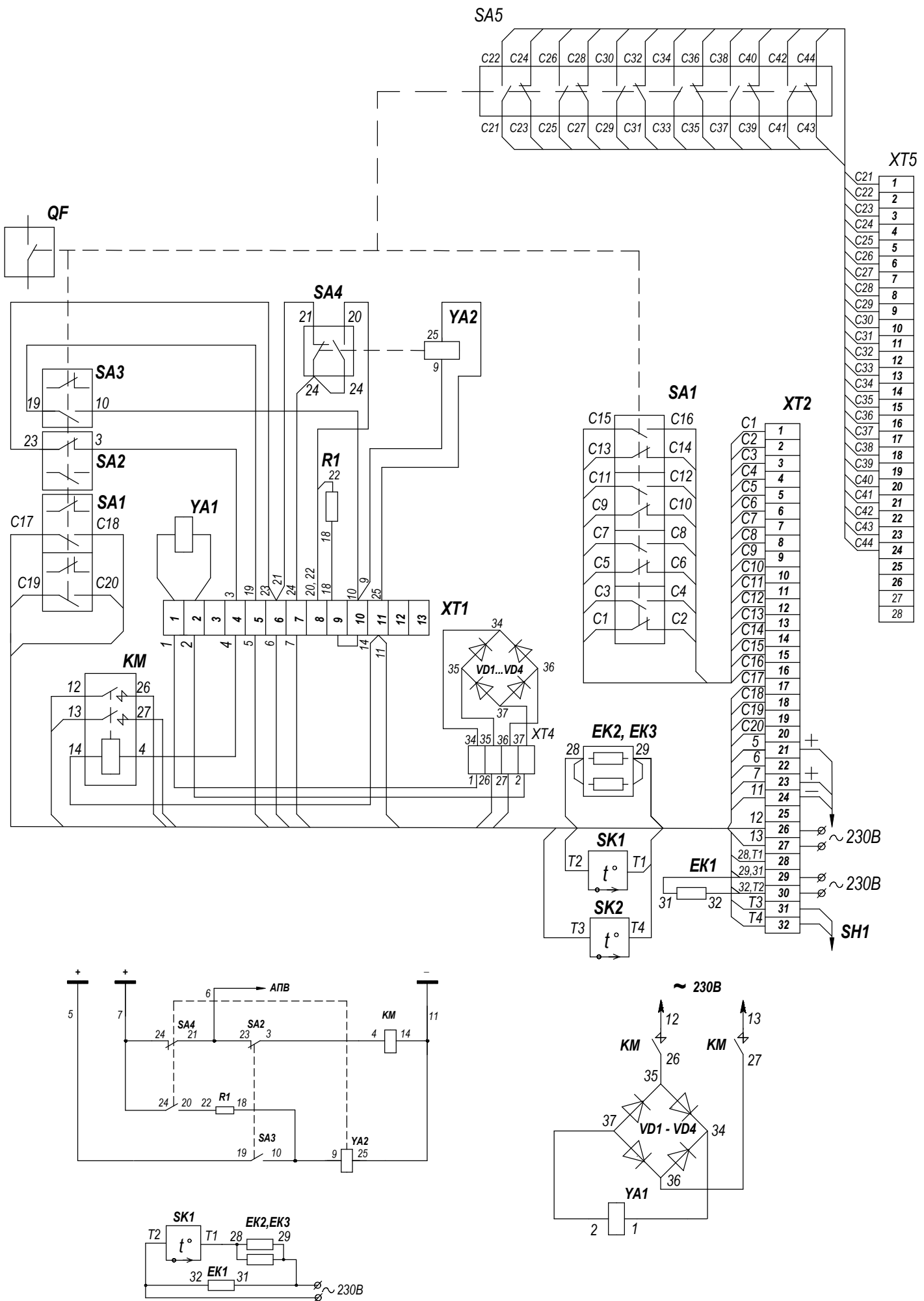
Рисунок 8. Схема электрическая соединений и принципиальная привода ПЭМ-УЭТМ ® -2 УХЛ1 с переключателем сигнальных контактов
