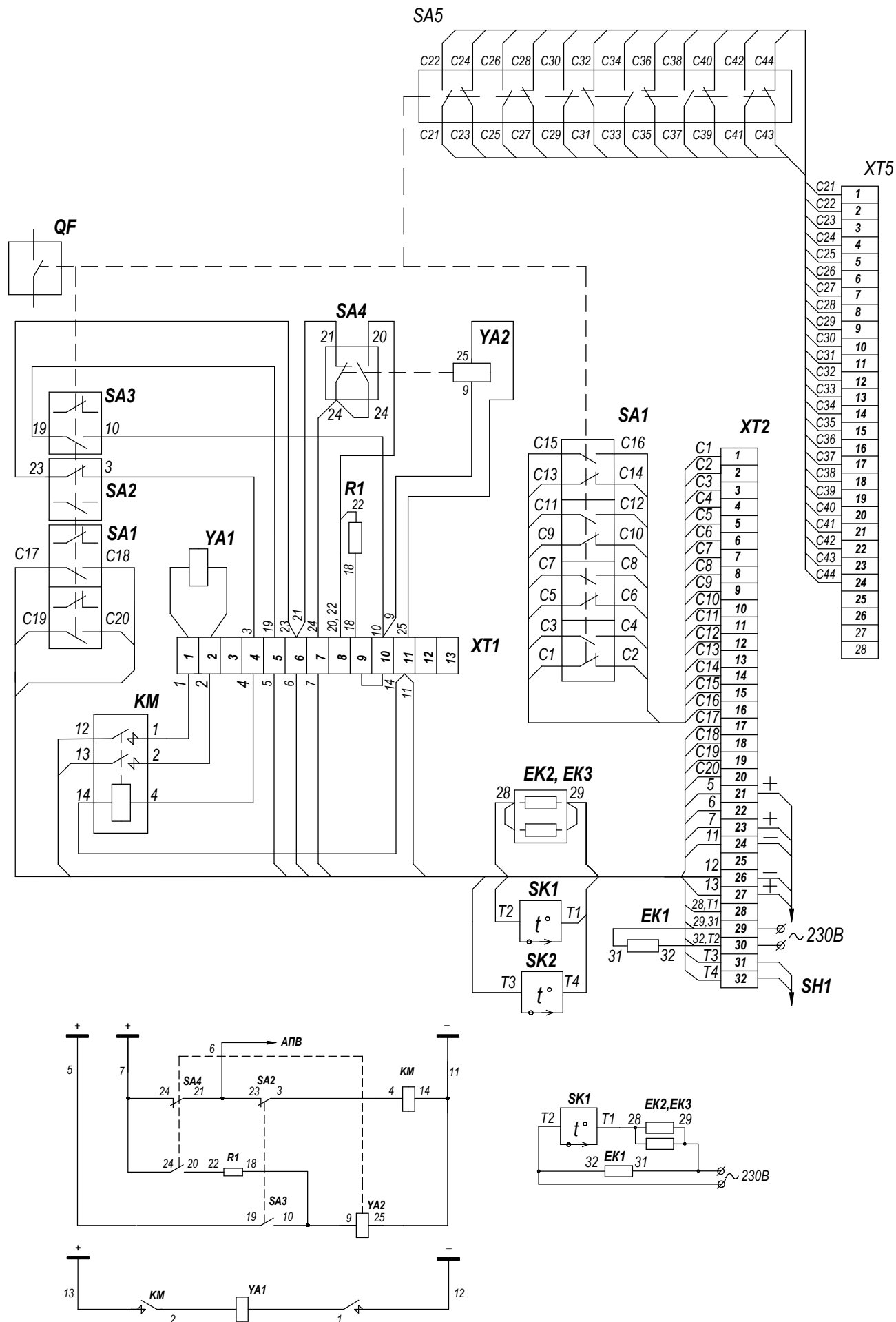
Рисунок 6. Схема электрическая соединений и принципиальная привода ПЭМ-УЭТМ®-1 УХЛ1 с переключателем сигнальных контактов
