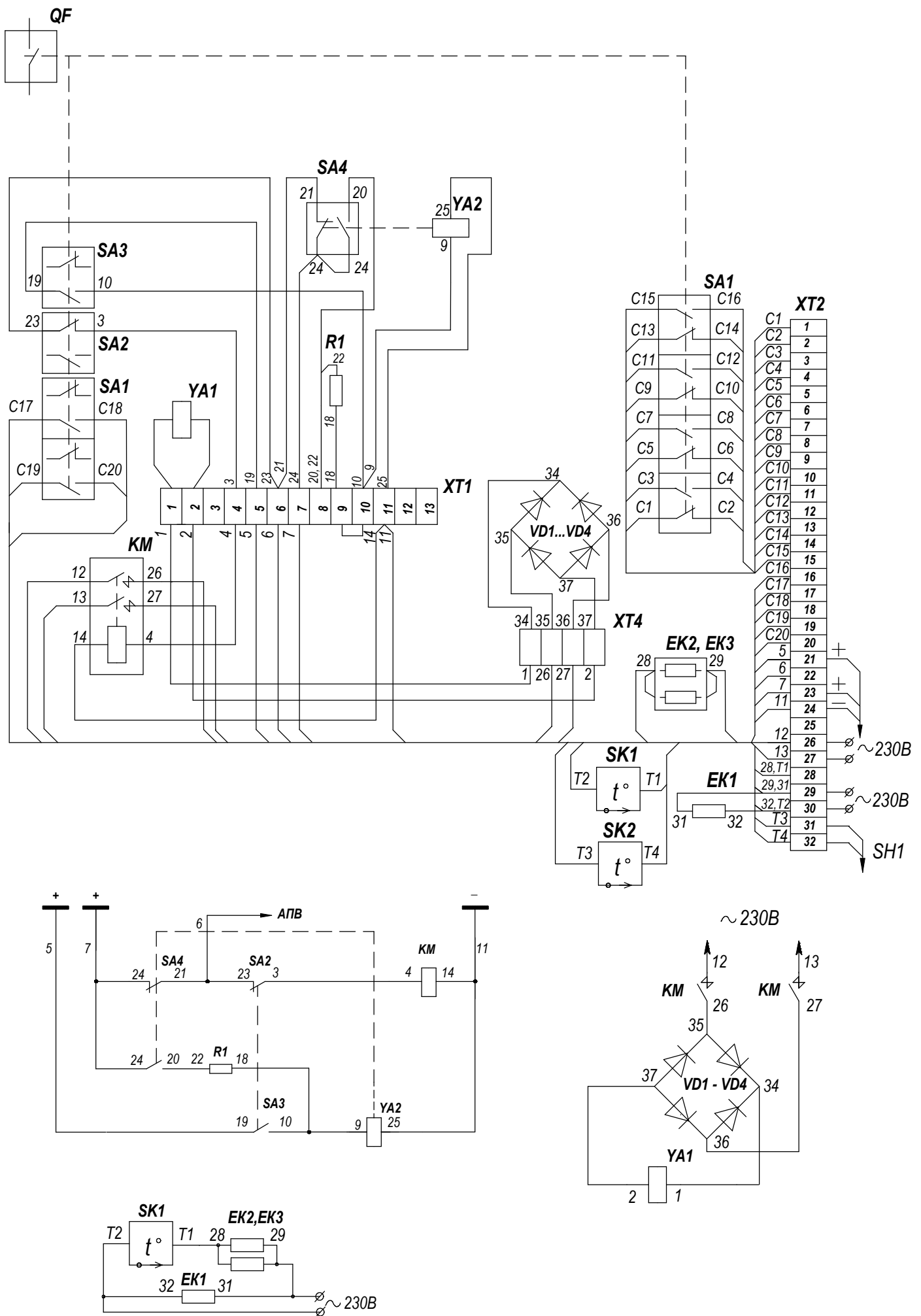
Рисунок 3. Схема электрическая соединений и принципиальная привода ПЭМ-УЭТМ®-2 УХЛ1
