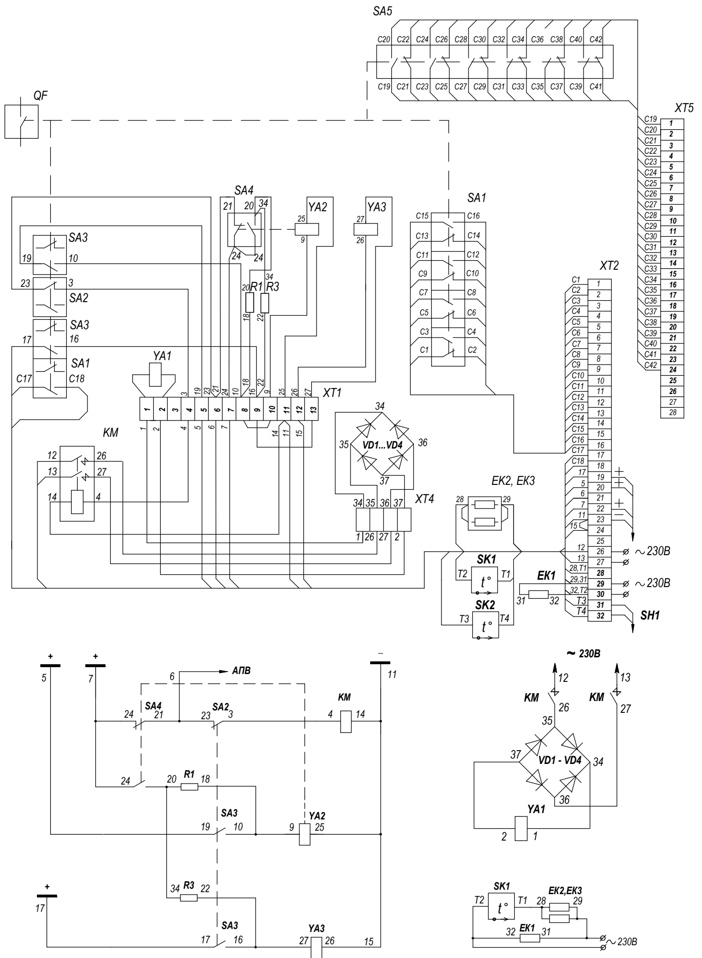
Рисунок 9. Схема электрическая соединений и принципиальная привода ПЭМ-УЭТМ ® -2 УХЛ1 с переключателем сигнальных контактов и двумя электромагнитами отключения
