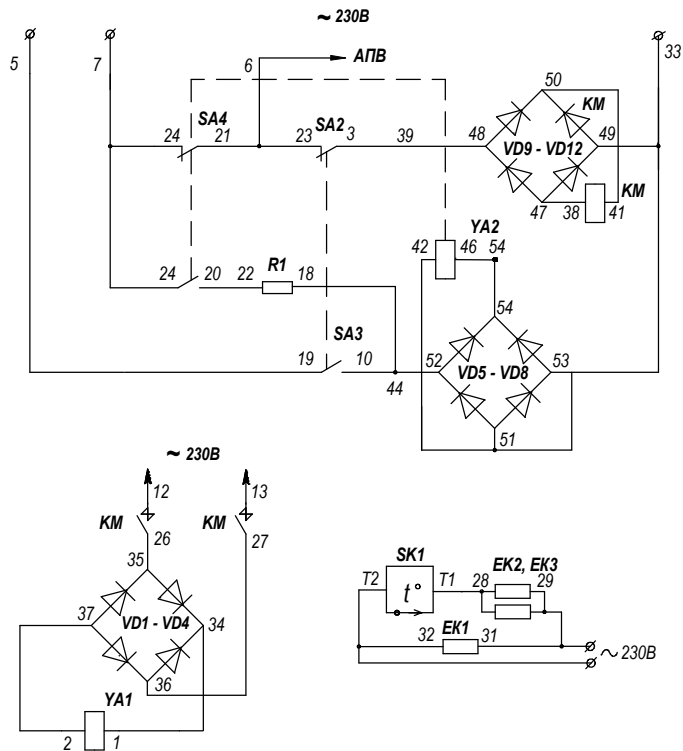
Рисунок 10. Схема электрическая соединений и принципиальная привода ПЭМ-УЭТМ®-3 УХЛ1 с переключателем сигнальных контактов
