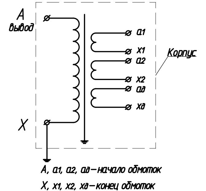
Схема обмоток трансформатора Первичная обмотка Вторичные обмотки
