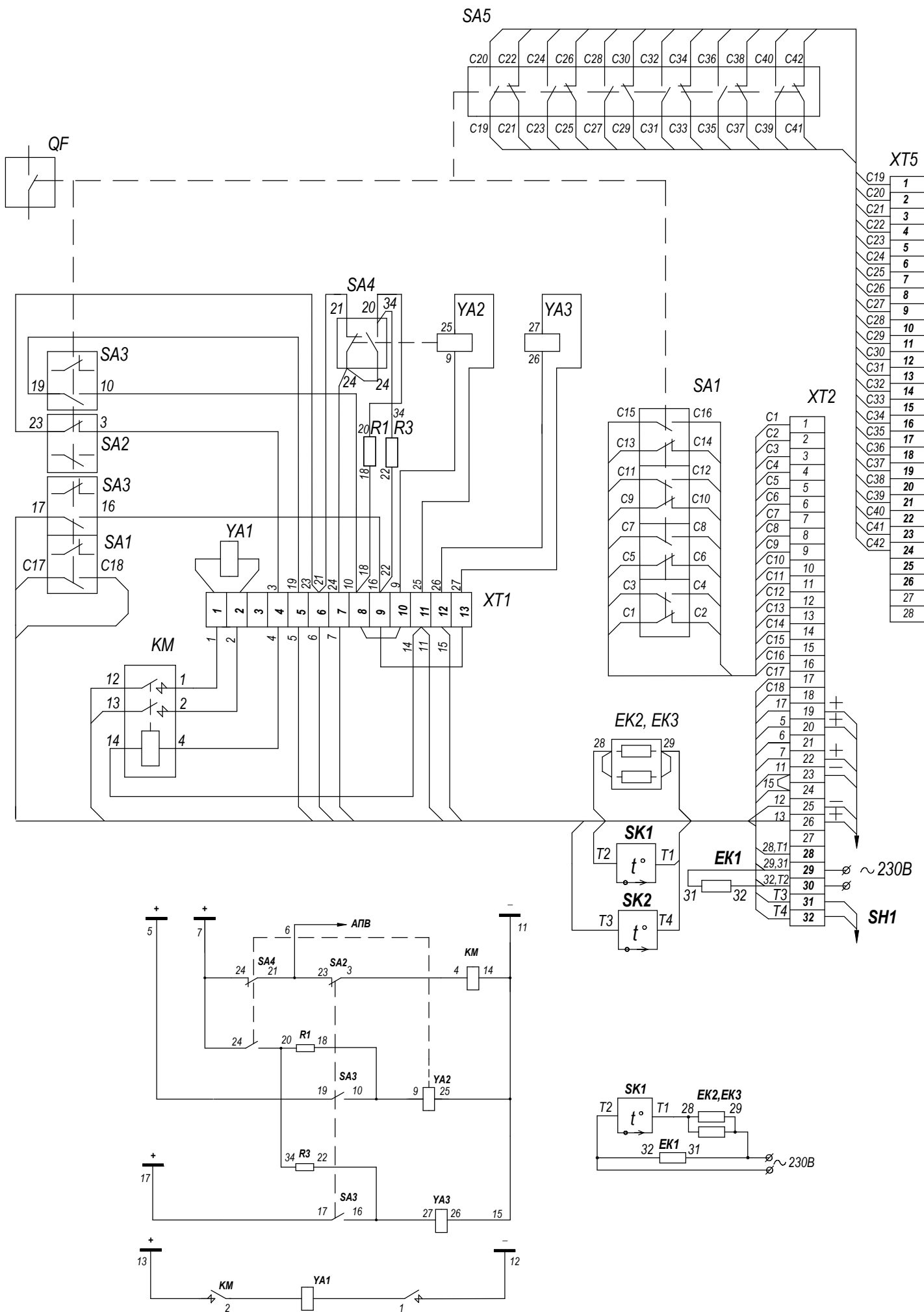
Рисунок 7. Схема электрическая соединений и принципиальная привода ПЭМ-УЭТМ®-1 УХЛ1 с переключателем сигнальных контактов и двумя электромагнитами отключения
